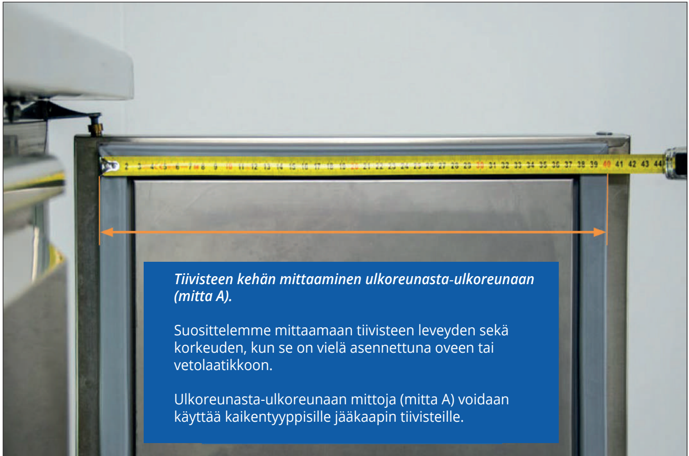
Mitta A Tiiviste en keh ä ulkoreunasta ulkoreunaan
