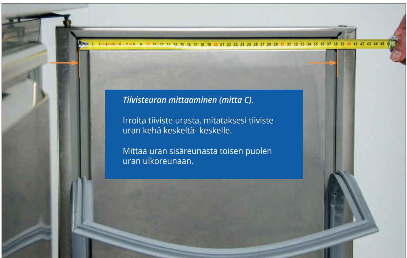
Mitta C Tiiviste uran keh ä keskelt ä keskelle
